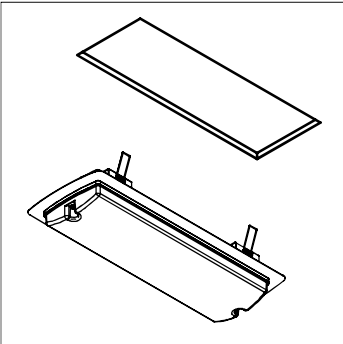
Inbouw (Optioneel - Niet inclusief) Zaagmaat 355x125mm
